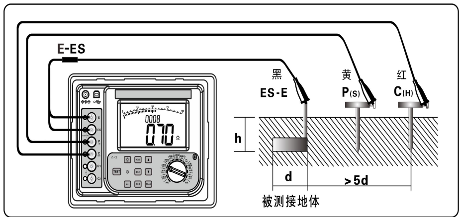
图 7（三线测试接地电阻示意图）
