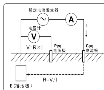
图 1 (接地测量原理图)
