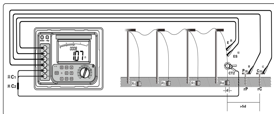
图 13 (四线选择法测试示意图)
