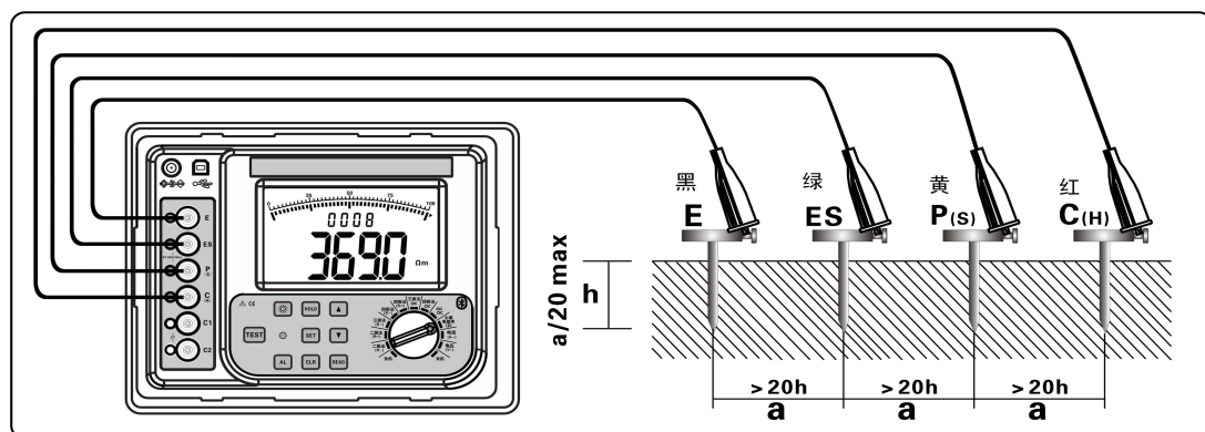
图 16 (土壤电阻率测试示意图)
