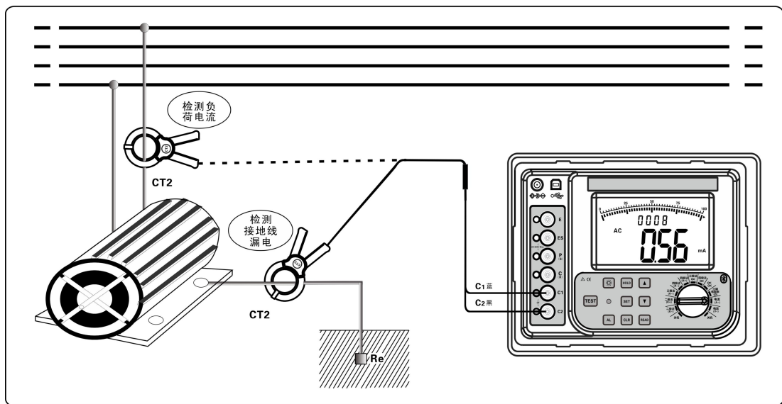
图 19（直流电阻测试示意图）
