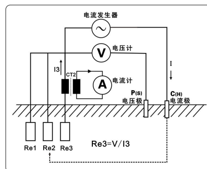
图 2 (选择法测量原理图)
