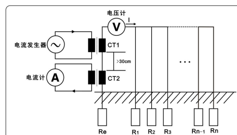
图 3 (双钳法测量原理图)
