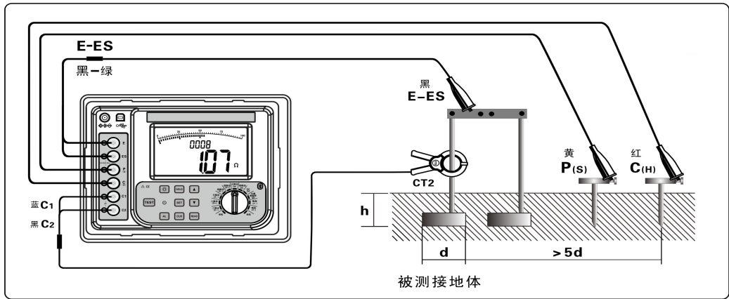
图 14（单钳三线选择法测试示意图）
