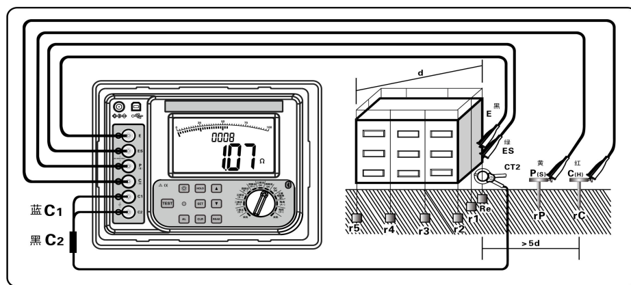
图 12 (四线选择法测试示意图)
