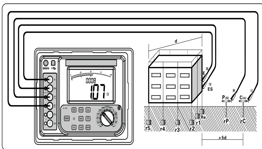
图 9（四线测试接地电阻示意图）
