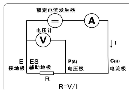
图 5 (直流电阻测试原理图)
