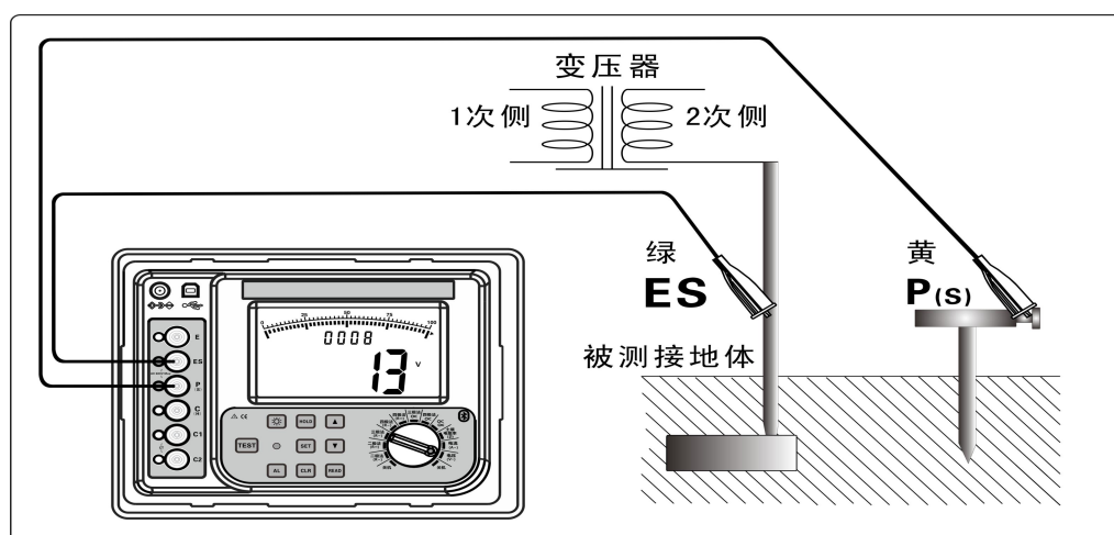
图 20（接地电压测试示意图）
